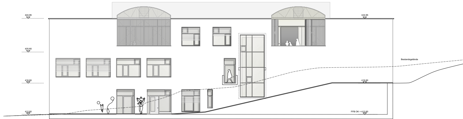
Ansicht Nord M 1:100
